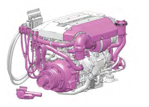
Kit de cambio de motores D3. Se incluyen todos los componentes necesarios, como un anillo adaptador, elevador de escape, pantalla térmica para el turbo y el elevador, cubierta del motor, instrucciones de instalación, etc.
