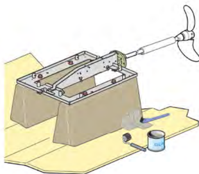
Ejemplo del manual de instalación de cómo reconstruir la bancada del motor
