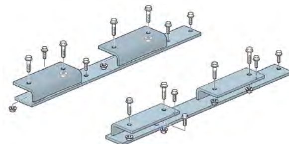
Ejemplo de componentes del kit (kit 23059553)
